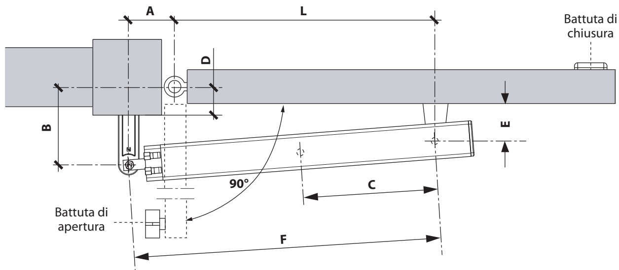
Quote di installazione in (mm) per apertura di 90°
